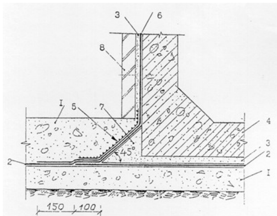
Рис. 17. Сопряжение гидроизоляции горизонтальной (наклонной) и вертикальной поверхностей
