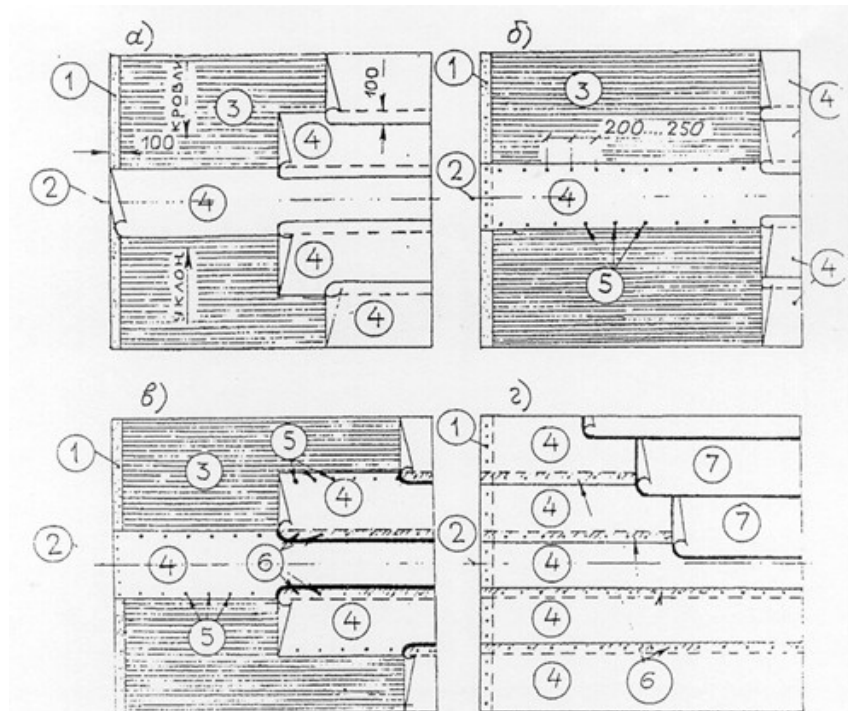
Рис. 14. Пример раскладки рулонных материалов при устройстве кровельного ковра с механическим закреплением нижнего слоя
