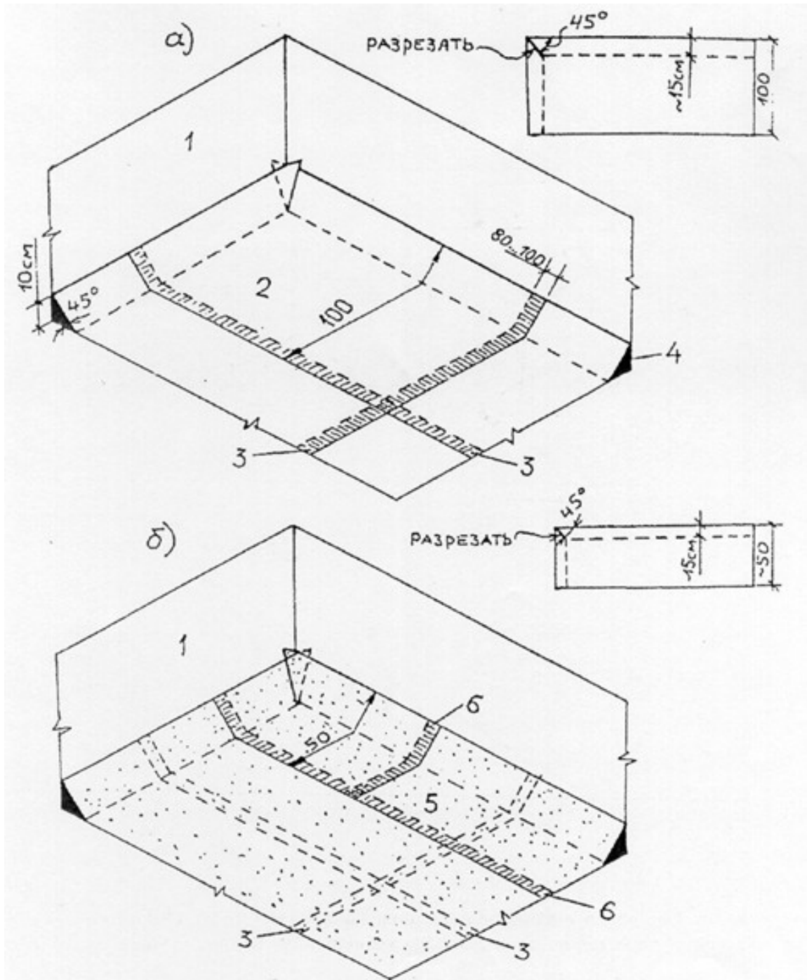
Рис. 5. Раскладка и раскрой полотнищ наплавляемого рулонного материала (а - нижнего слоя; б — верхнего слоя) при устройстве основного кровельного ковра в углу парапета 1 - парапет; 2 - нижний слой ковра; 3 - нахлестка полотнищ нижнего слоя; 4 - наклонный переходный бортик; 5 - верхний слой ковра (с крупнозернистой посыпкой); 6 - нахлестка полотнищ верхнего слоя.
