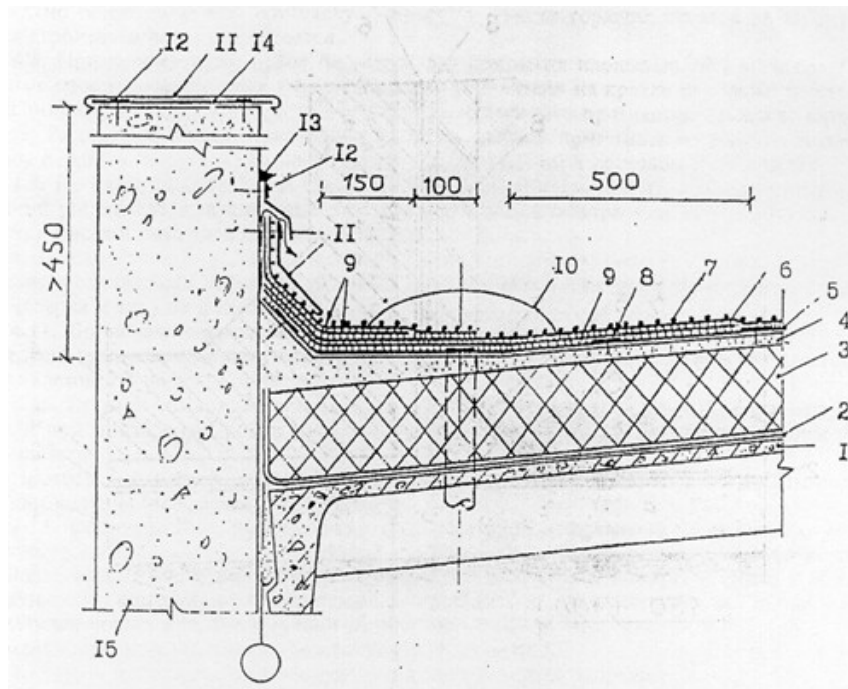
Рис. 16. Примыкание кровли к парапету высотой более 450 мм
