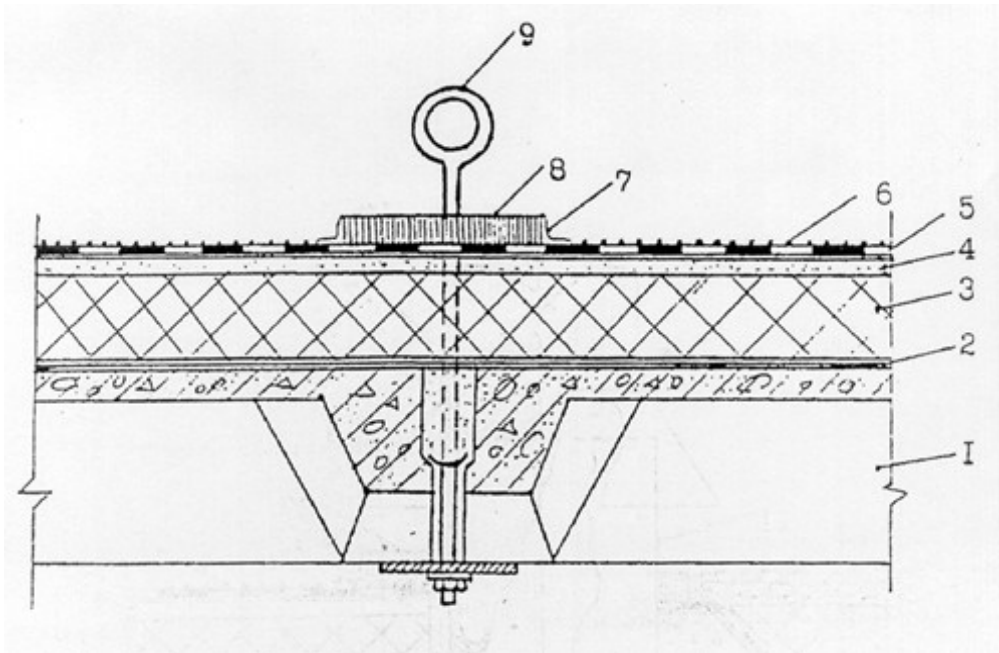
Рис. 10, Пропуск анкера через кровельный ковер
