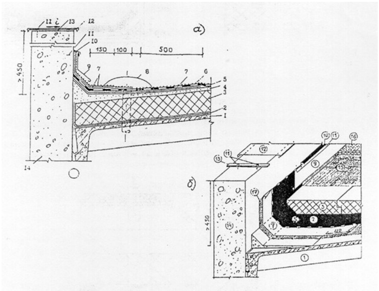
Рис. 4. Примыкание кровли к парапету высотой более 450 мм
