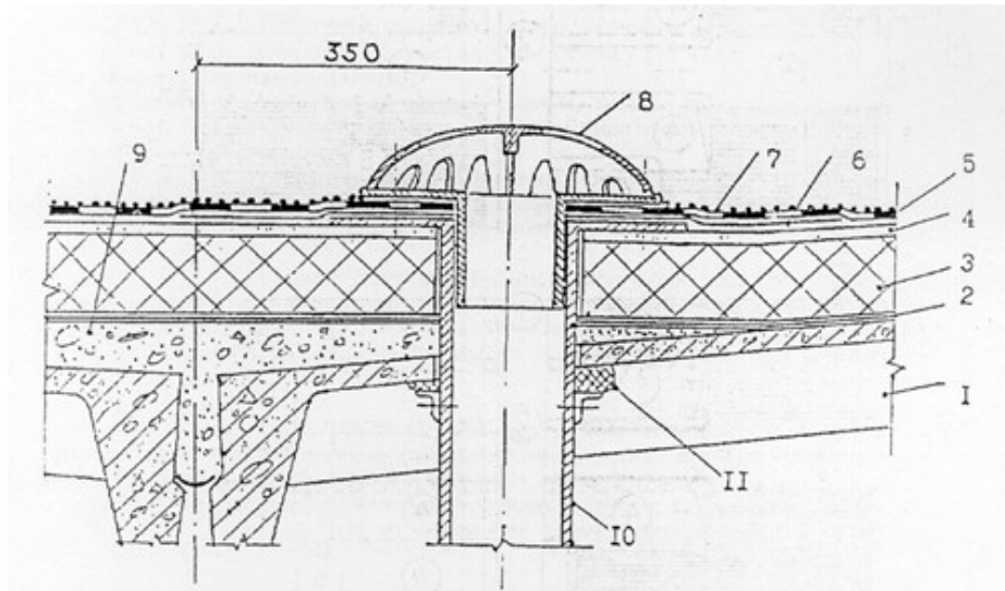
Рис. 13. Воронка внутреннего водостока
