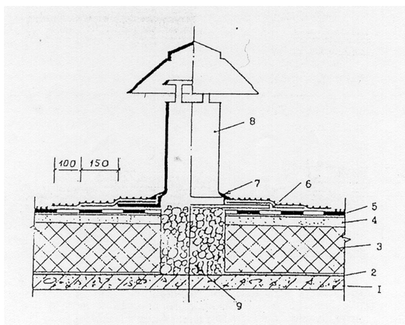
Рис. 1. Вентиляционный патрубок
