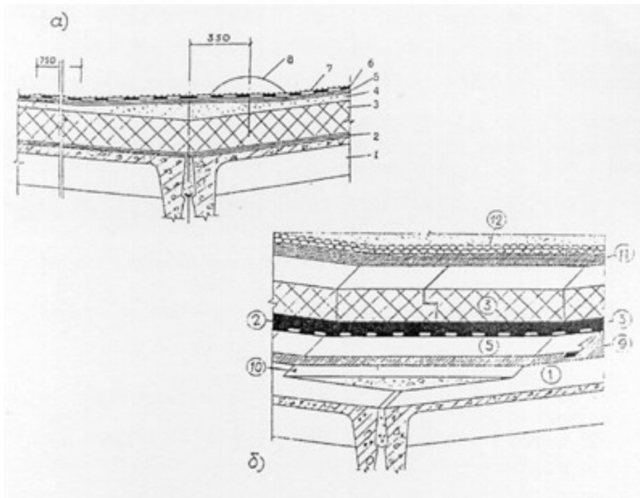
Рис. 8. Ендова кровли
