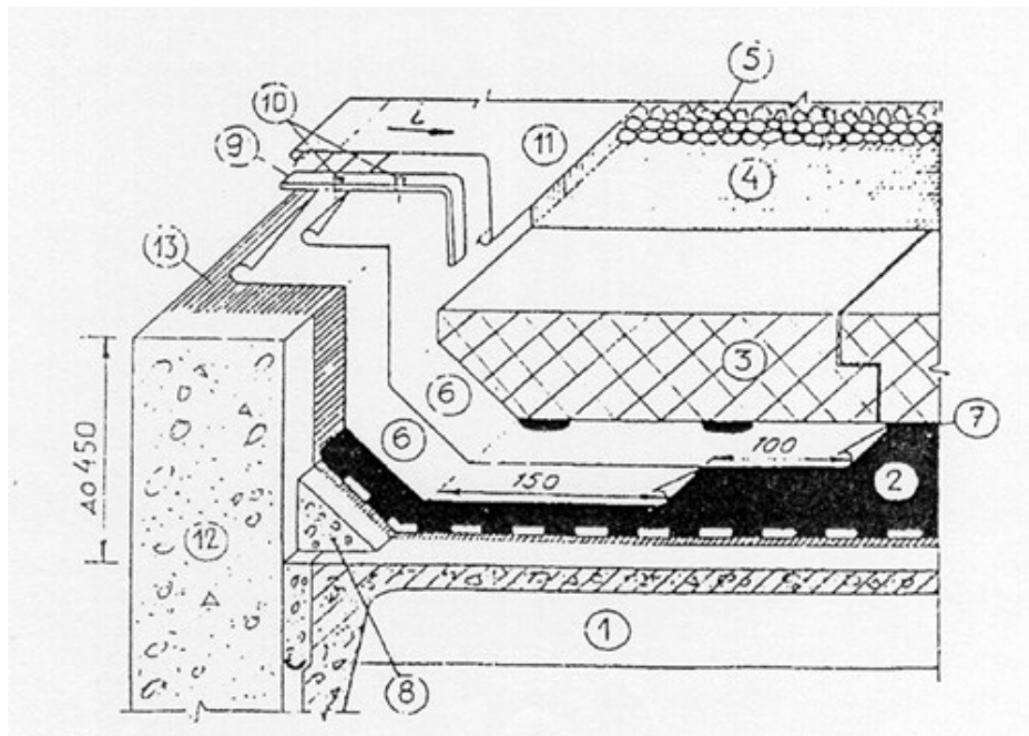
Рис.3. Примыкание инверсионного покрытия к парапету высотой до 450мм
