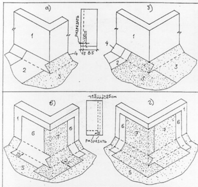
Рис. 12. Раскладка и раскрой полотнищ наплавляемого рулонного материала при устройстве кровельного ковра (а и б - основного, в и г - дополнительного) на поверхности внешнего угла, например: вентиляхты
