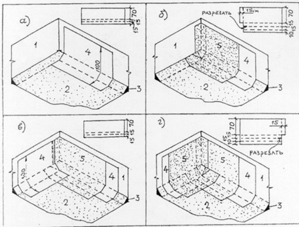
Рис.6. Раскладка и раскрой полотнищ наплавляемого рулонного материала при устройстве дополнительного кровельного ковра в углу парапета 1 - парапет; 2 - основной кровельный ковер; 3 - переходный наклонный бортик; 4 - нижний слой дополнительного ковра; 5 - верхний слой (с крупнозернистой по сыпкой) дополнительного ковра.
