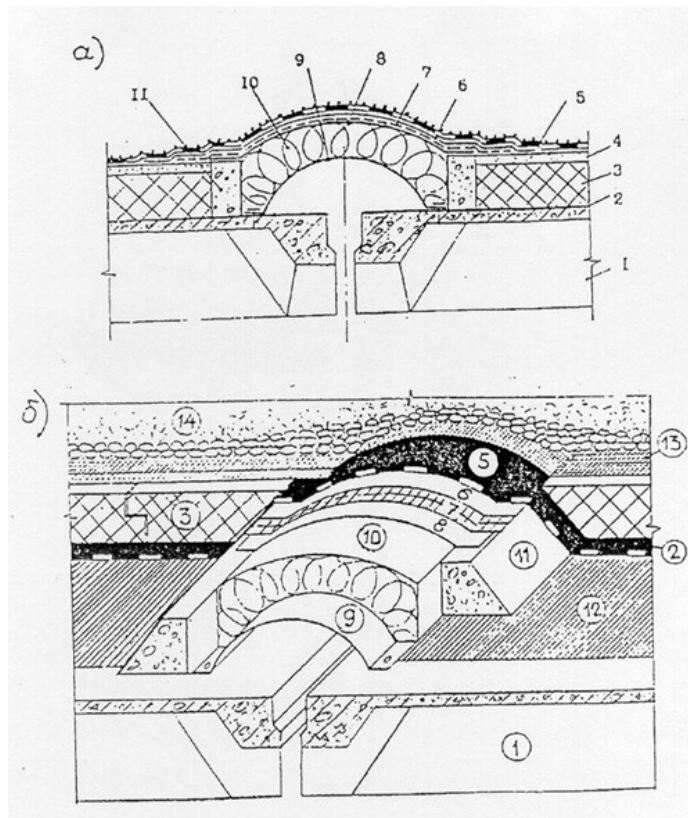
Рис. 11. Деформационный шов в покрытии
