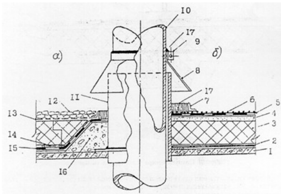
Рис. 9. Примыкание кровли к трубе
