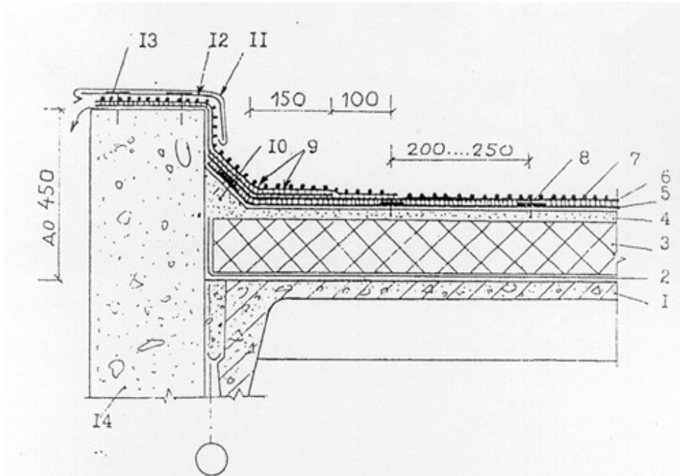
Рис. 15. Примыкание кровли к парапету высотой до 450 мм
